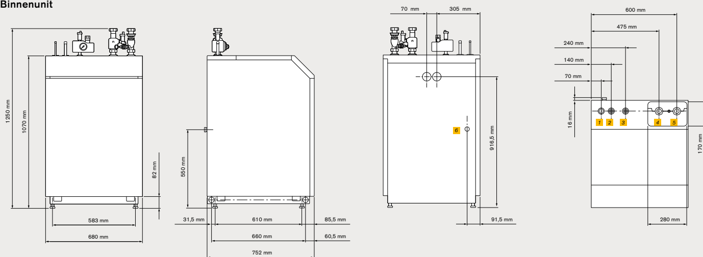
Binnenunit
