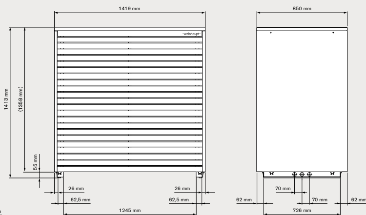
WBB 20 buitenunit
