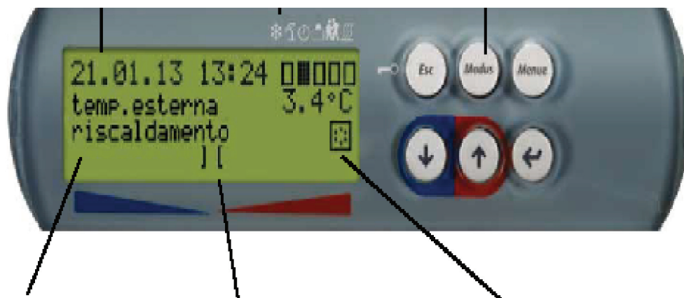
Fig. 4.2: Programmatore della pompa di calore con schermo standard a display LCD integrato con tasti di comando
