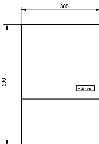
Afb. 3.1: Afmetingen van de aan de wand gemonteerde cascaderregelaar
