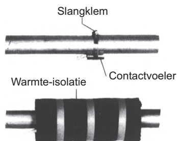
Afb. 3.4: Montage van een buiscontactvoeler
