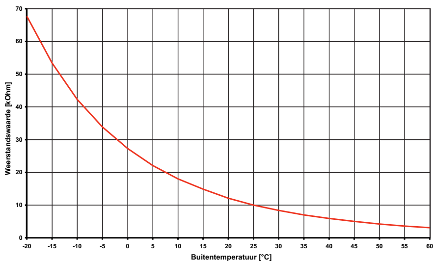
Afb. 3.3: Voelercurve NTC-10 voor de aansluiting op de verwarmingsregelaar
