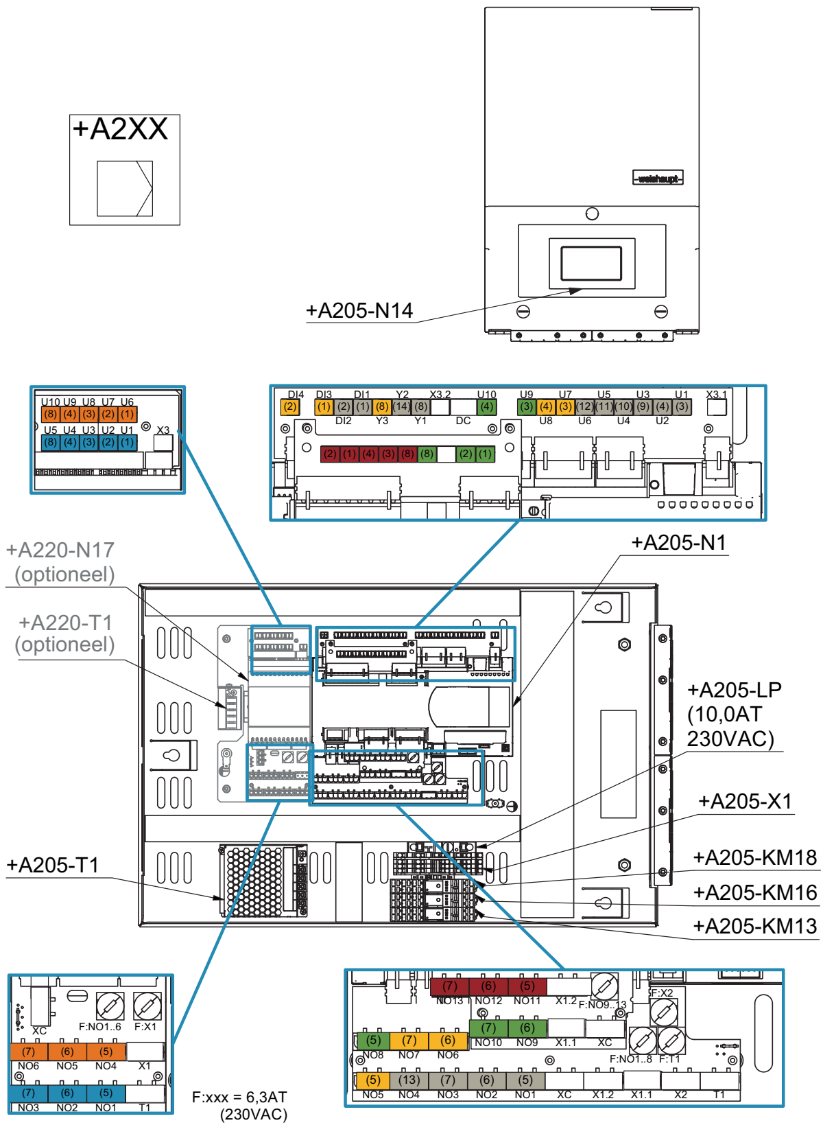
Afb. 4.1: Aan de wand gemonteerde cascadereregelaar
