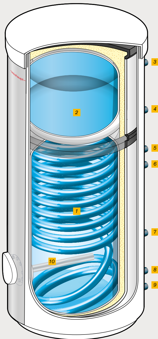
Weishaupt modularni hranilnik WMS
