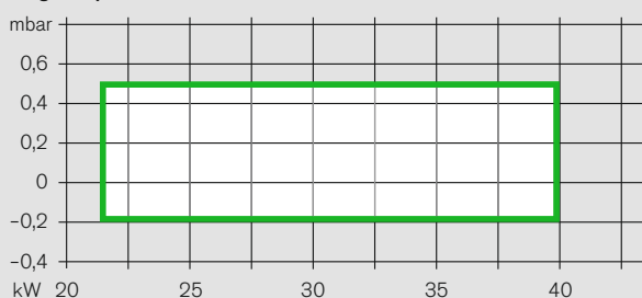
Plage de puissance WL5/1-B LN-BE
