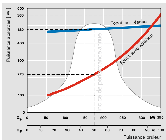
Réduction de la puissance absorbée, exemple brûleur gaz WG 30
