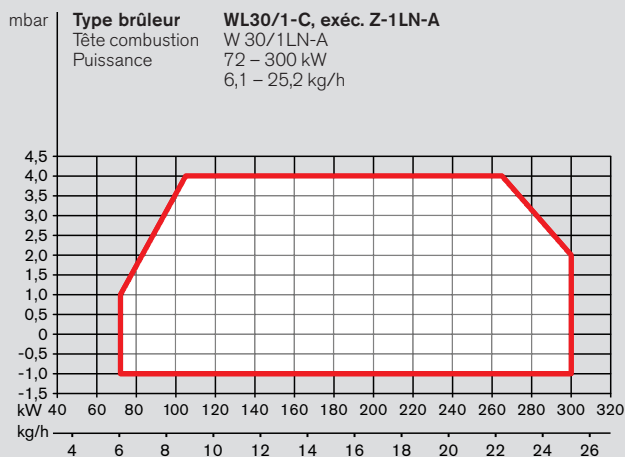
Plage de puissance WL30/1C, exéc. Z-1LN-A
