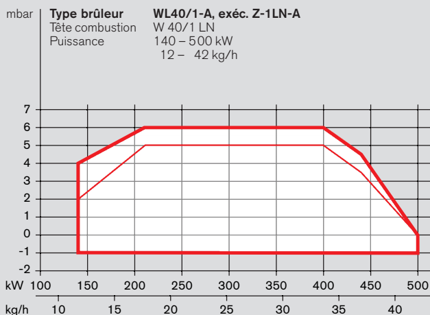
Plage de puissance WL40/1A, exéc. Z-1LN-A
